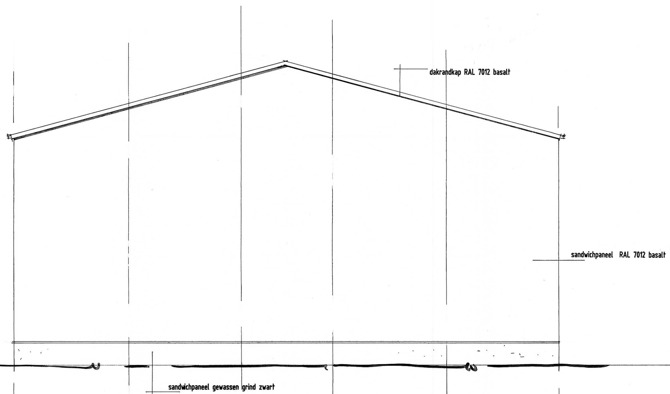
L. ZIJGEVEL
